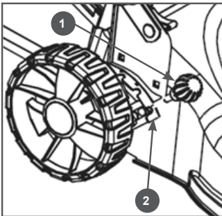
Рис. 8 Регулировка высоты кошения 1. Рычаг 2. Сектор регулятора
