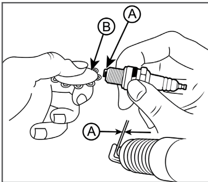
Рис. 13 Обслуживание свечи зажигания А-зазор, В-щуп
