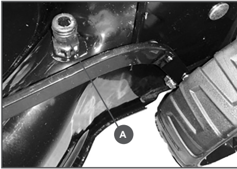
Рис. 14 Расположение коннектора для подключения шланга А - коннектор
